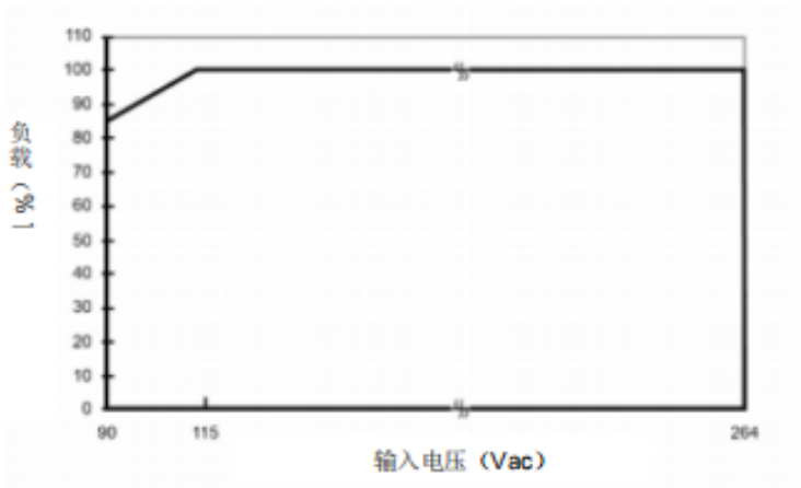
图 2 ) AC 输入电压降额_ 输出负载降额对应输入电压
