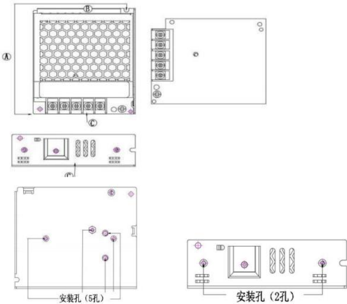
图. 3.2 安装位置
