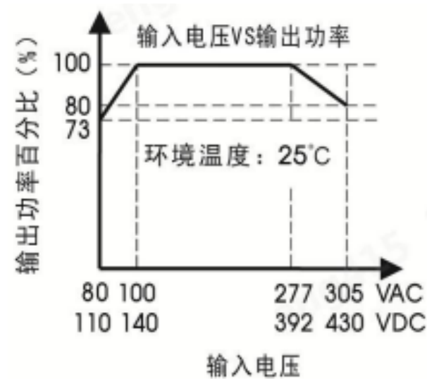
图 2 ) AC 输入电压降额_ 输出负载降额对应输入电压
