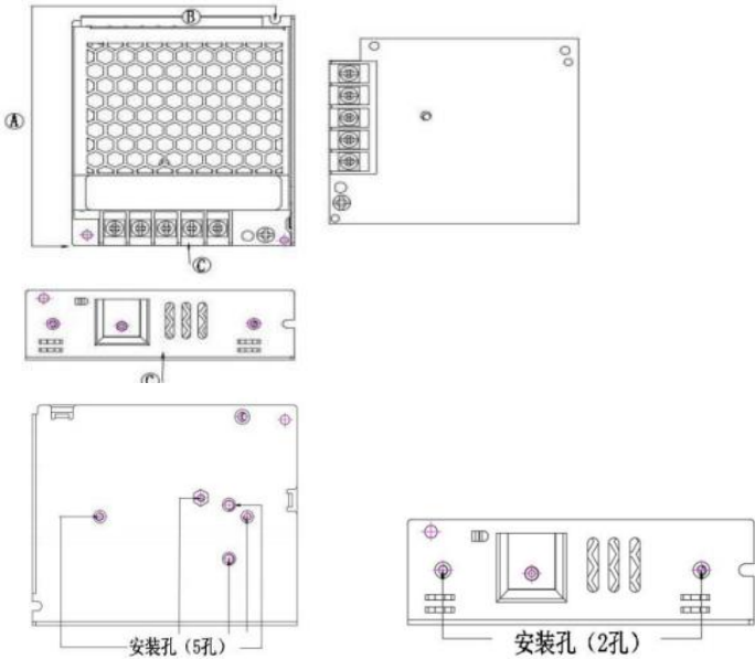
图. 3.2 安装位置
