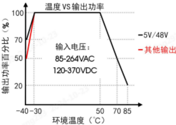
图 2 ) AC 输入电压降额_ 输出负载降额对应输入电压
